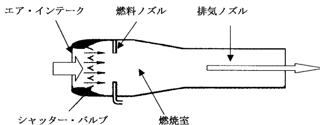
図2-3 パルス・ジェット
