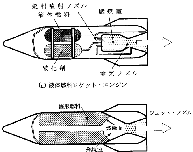
(b) 固体燃料ロケット・エンジン
