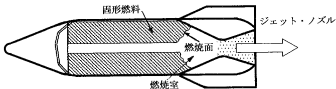
(b) 固体燃料ロケット・エンジン
